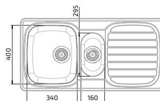
Insatsbänk Granberg ES30 - 76,6 cm
